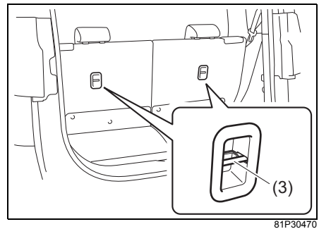
(3) テザーアンカー
